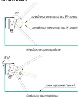
Рис.5 Пример установки извещателя
