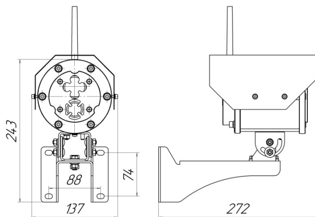
Рисунок 2.3 Монтажные размеры «C2000P-Spektron-609-Exd-A»
