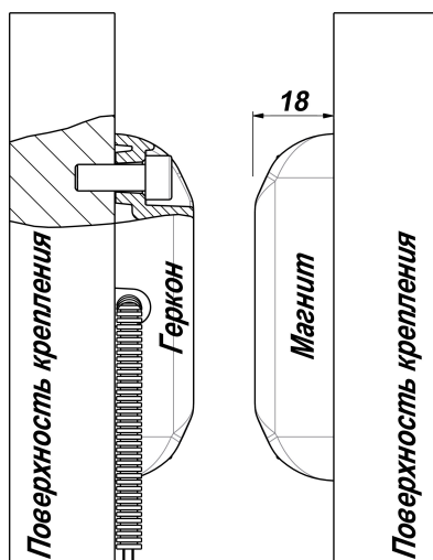
Рис. 2. Совмещение задающего и исполнительного блоков.
