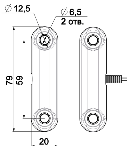
Рис. 1. Габаритные и установочные размеры: исполнительный блок –79x20x18. задающий блок –79x20x18.
