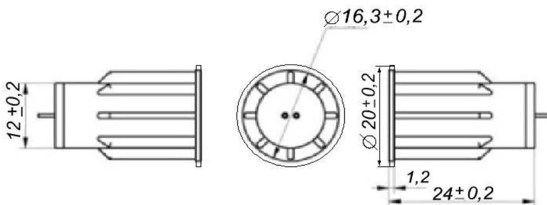
рис.1. Габаритные и установочные размеры
