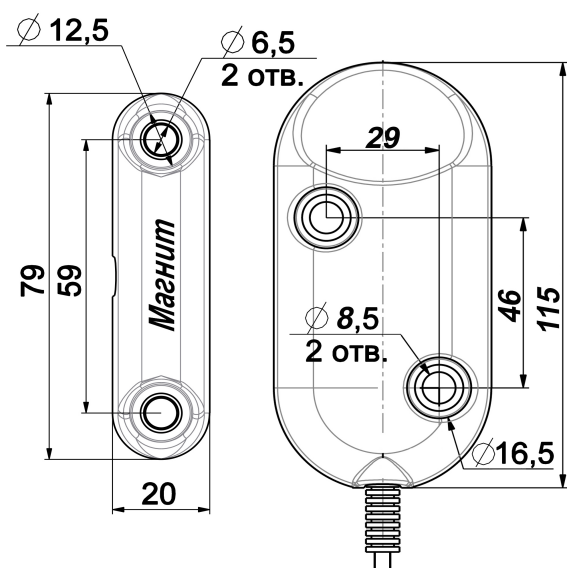
Рис.1. Габаритные и установочные размеры: исполнительного задающий и исполнительный блоки -115x56x14.
