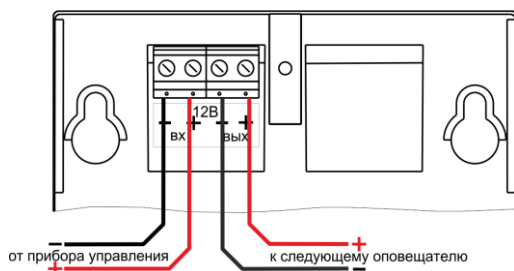
Рис.2 Схема подключения оповещателя
