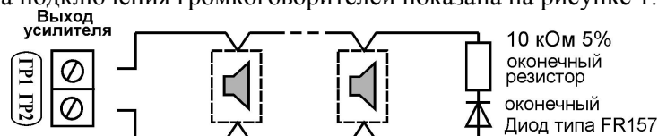
Рисунок 1. Схема подключения громкоговорителей
