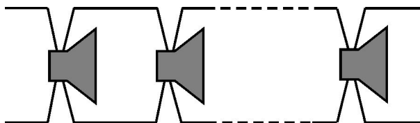
Рисунок 8. Схема подключения громкоговорителей на «проход»
