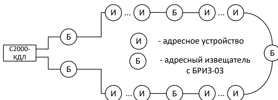
Рисунок 2.2.3 Топология «кольцо»
