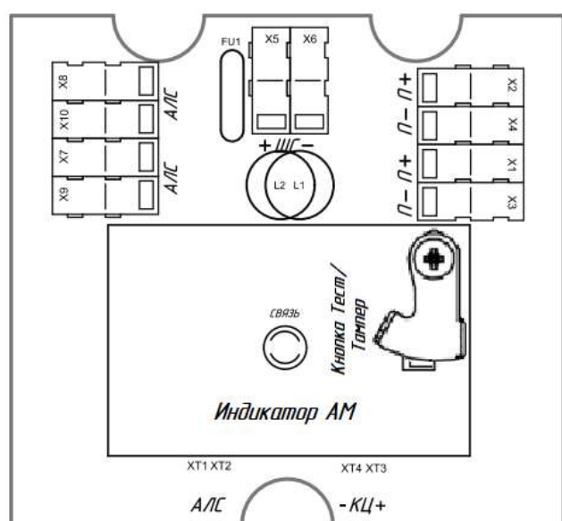
Рис. 6. Расположение монтажных клемм адресного модуля «МА Рубеж ОП».
