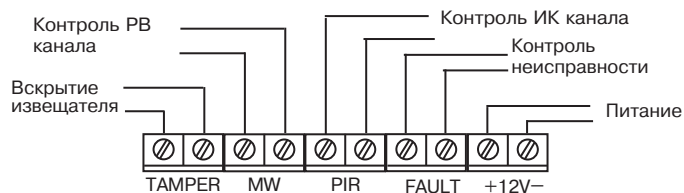
Рисунок 3 – Клеммы подключения
