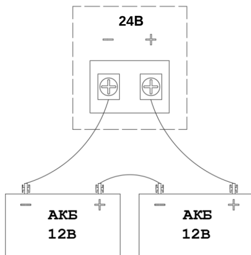
Рис. 3.1. Схема подключения АКБ к LPA-PRESTA-2
