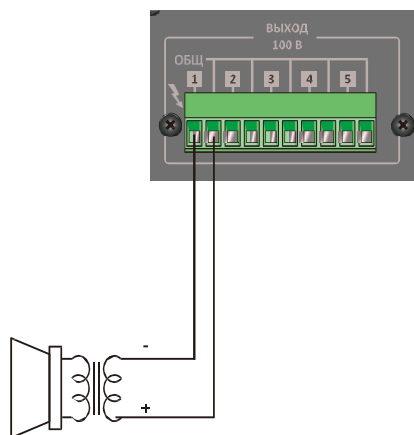
Рис. 2.2. Схема подключения громкоговорителей к LPA-TA-240MZ
