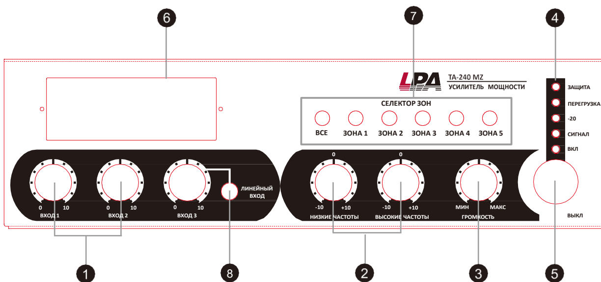
Рис. 3.1. Схема расположения средств управления LPA-TA-240MZ
