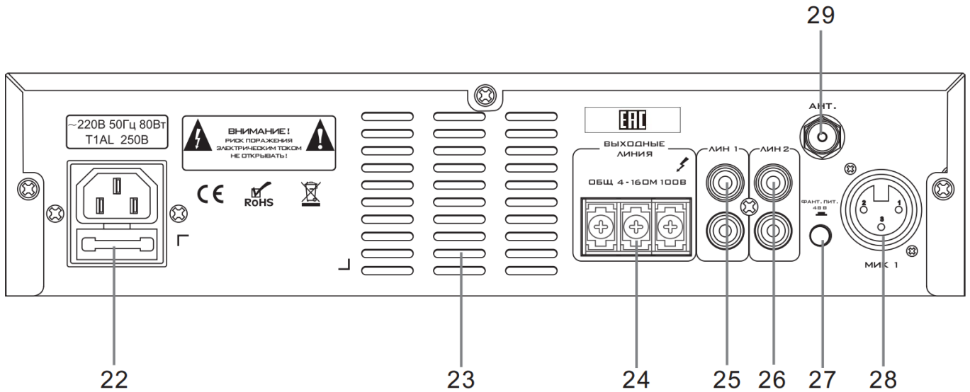
Рис. 3.3. Схема расположения средств управления LPA-TA-40M
