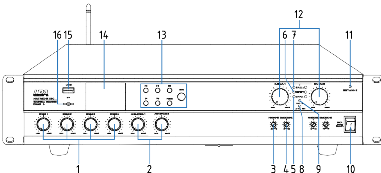
Рис.2.2. передняя панель
