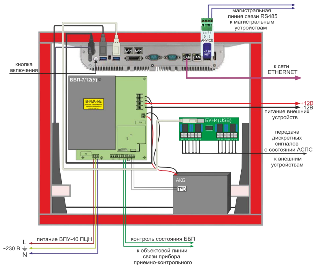
Рис.1. Устройство ВПУ-40 ПЦН
