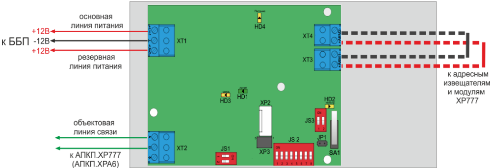
Рис. 1. Внешний вид платы модуля и схема подключений
