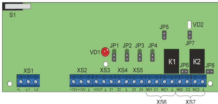
Рис. 2 Внешний вид платы МШ4-4
