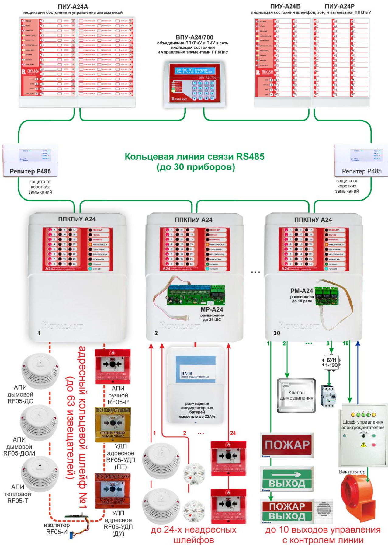
Рисунок 1. Структурная схема ППКПиУ и компонентов
