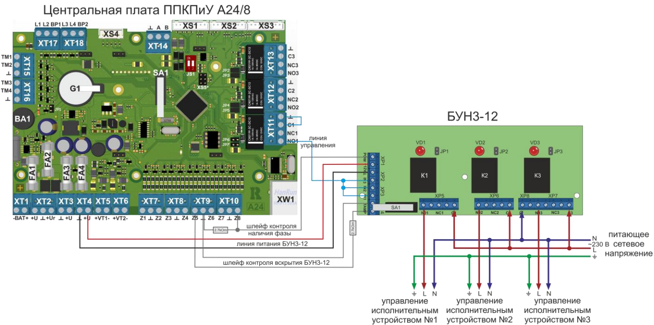
Рисунок 100. Схема подключения БУНЗ-12 к ППКПиУ А24/8.
