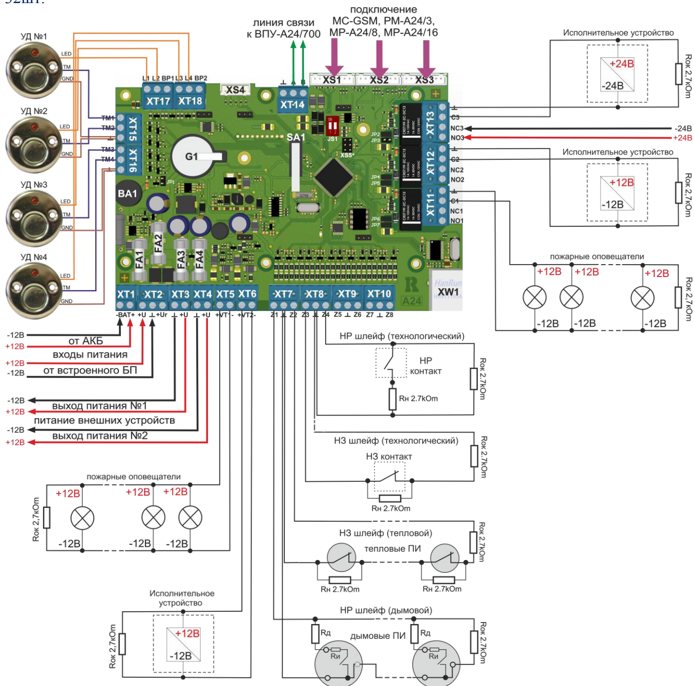
Рисунок 6. Схема подключения A24/8 с отключенной функцией «адресный шлейф»
