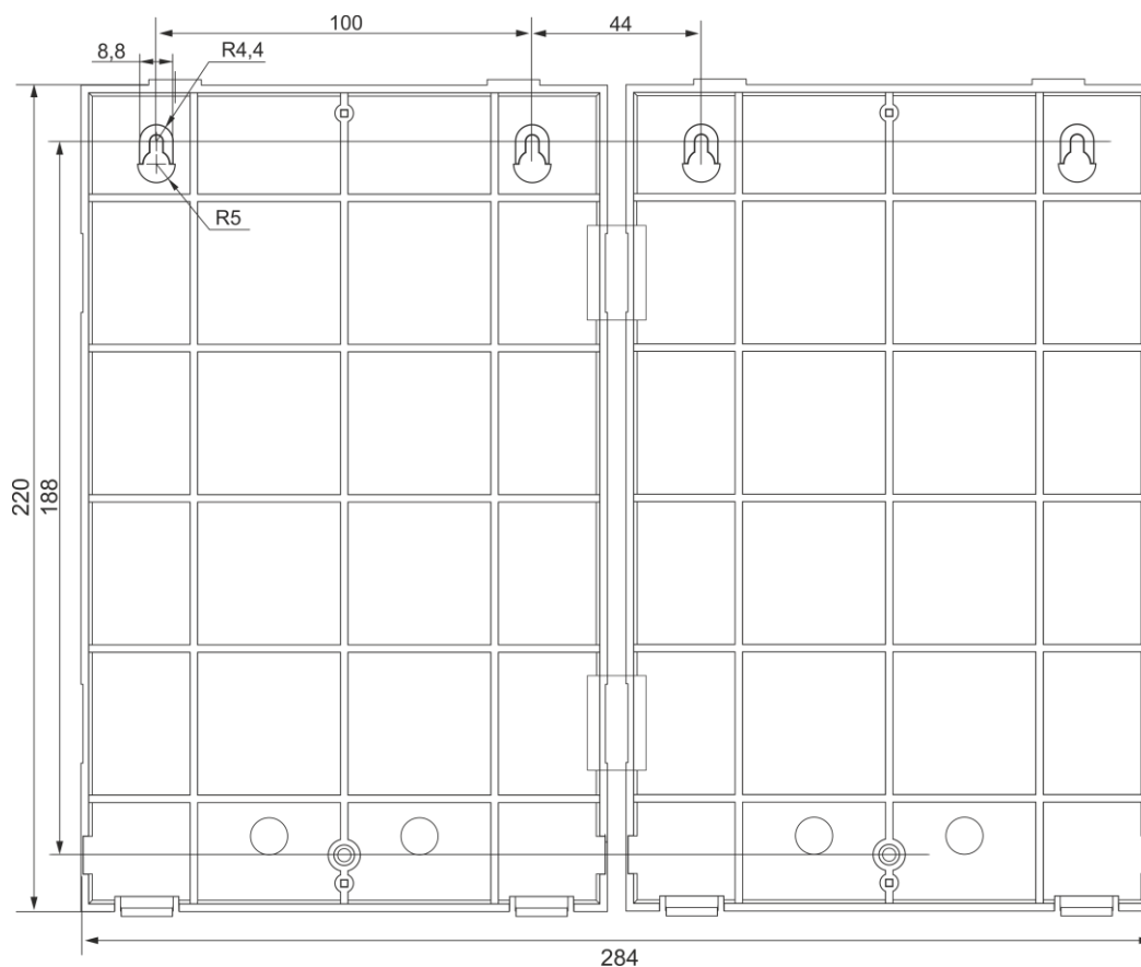
Рисунок 118. Установочный чертеж ПИУ-A24А или ПИУ-A24Б при применении совместно с одной ПИУ-A24Р
