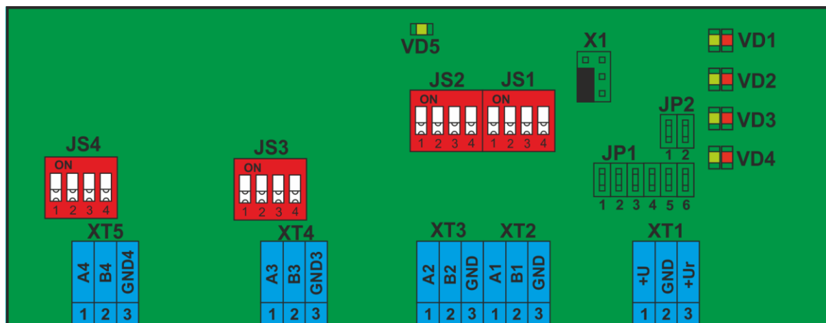
Рисунок 86. Внешний вид платы P485
