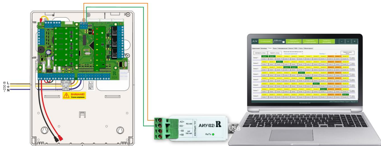
Рисунок 127. Схема подключения для конфигурирования ППКПиУ A24
