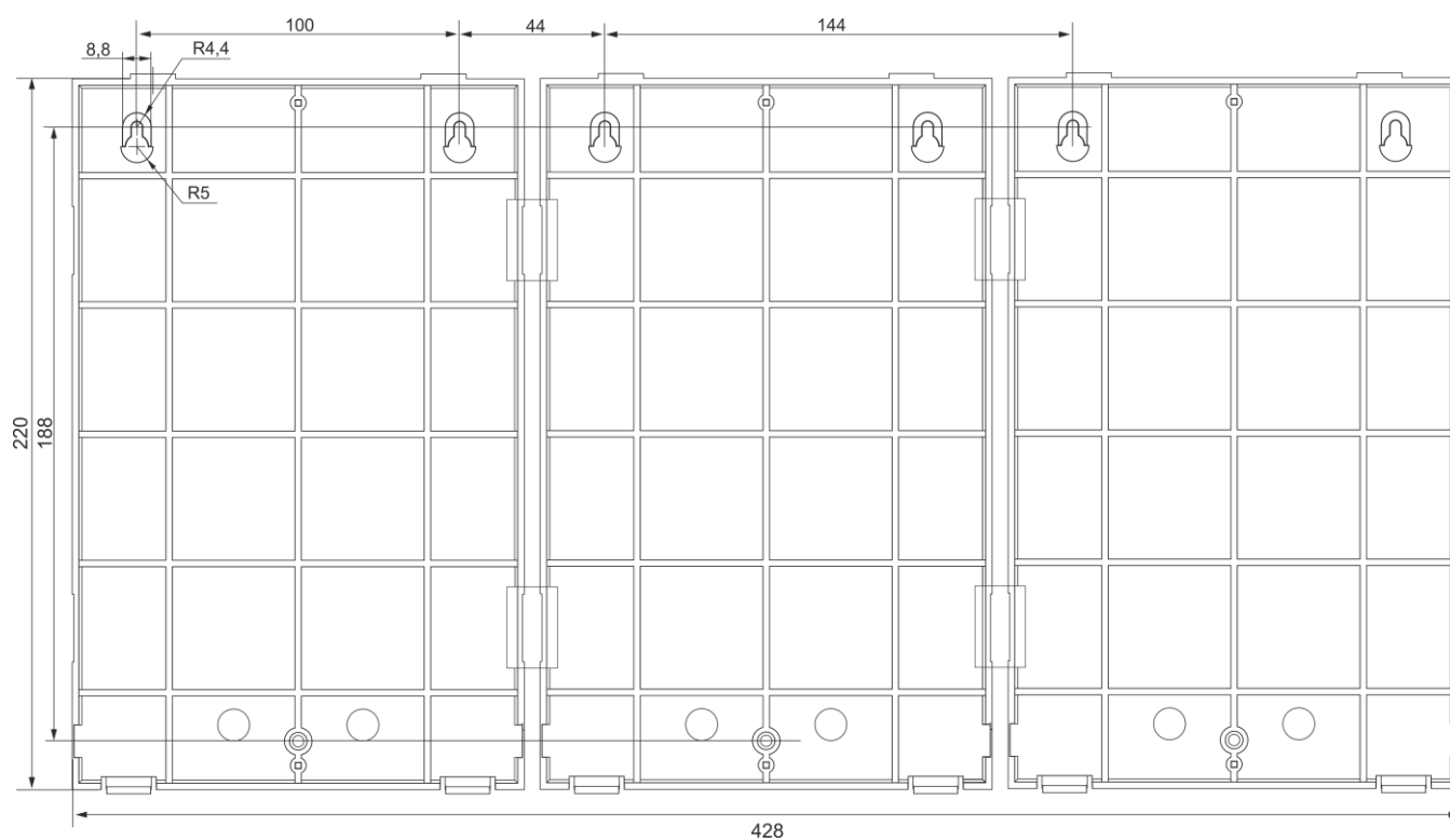
Рисунок 119. Установочный чертеж ПИУ-A24Б при применении совместно с двумя ПИУ-A24Р
