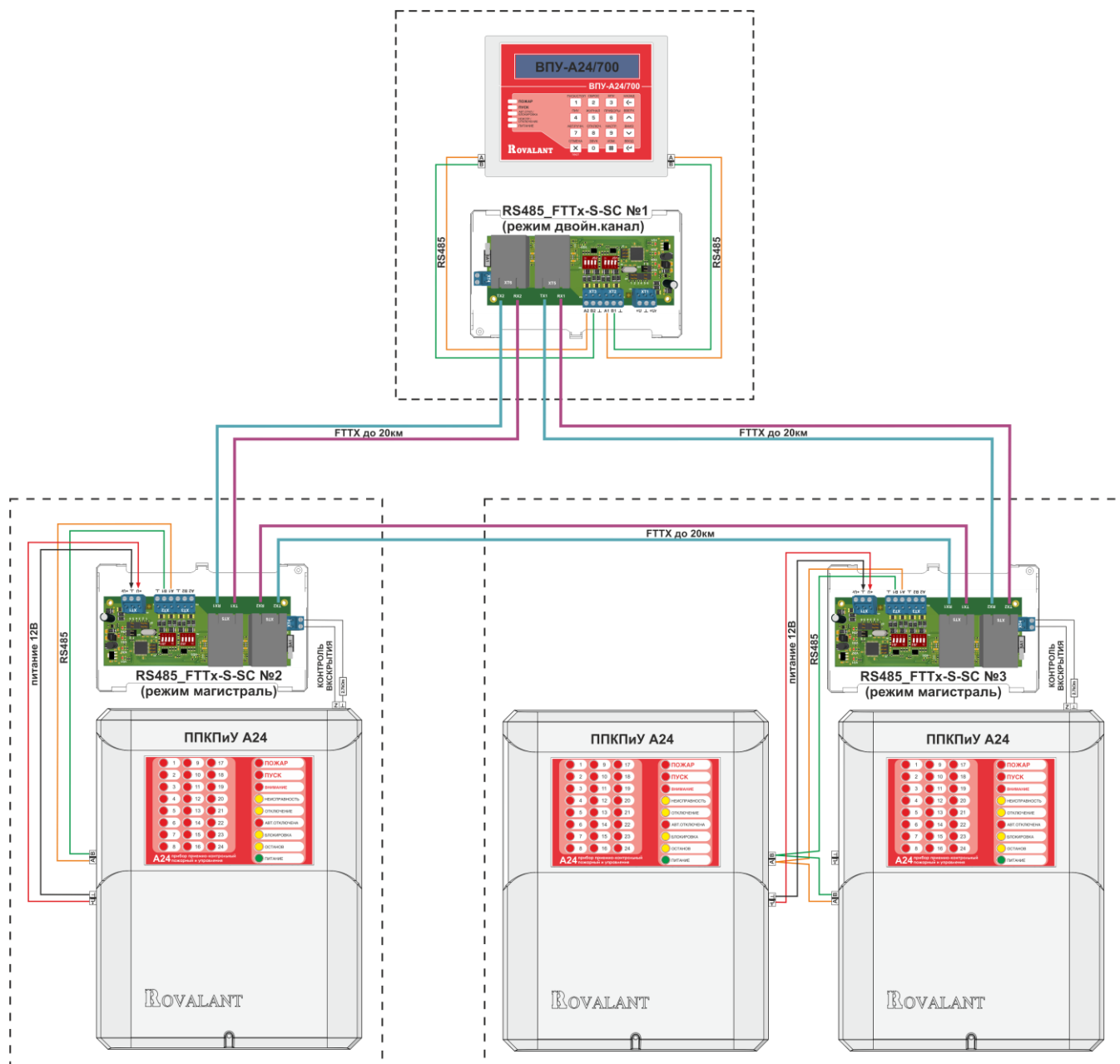
Рисунок 93. Схема организации оптоволоконной линии связи между ВПУ-А24/700 и приборами серии «А24»
