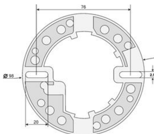
Рисунок 122. Установочный чертеж RF04-ДО, ИП101-02-ВМ, изолирующего основания ХР777
