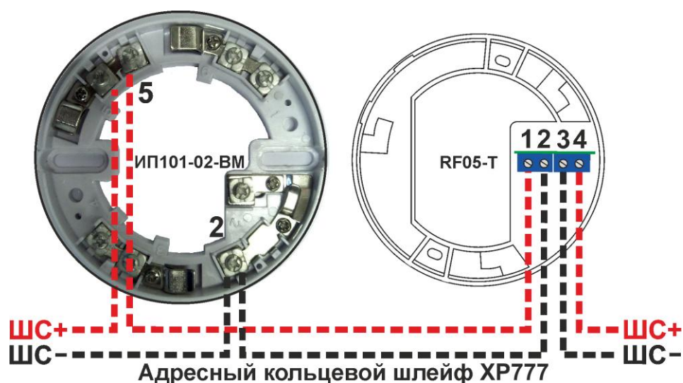
Рисунок 108. Схема подключения ИП101-02-ВМ, RF05-Т
