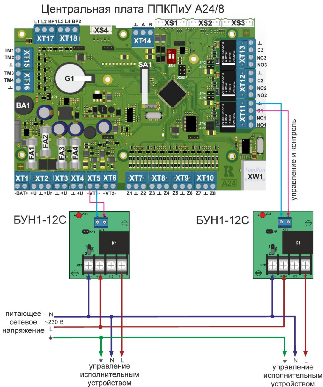
Рисунок 95. Схема подключения БУН1-12С к ППКПиУ А24/8.
