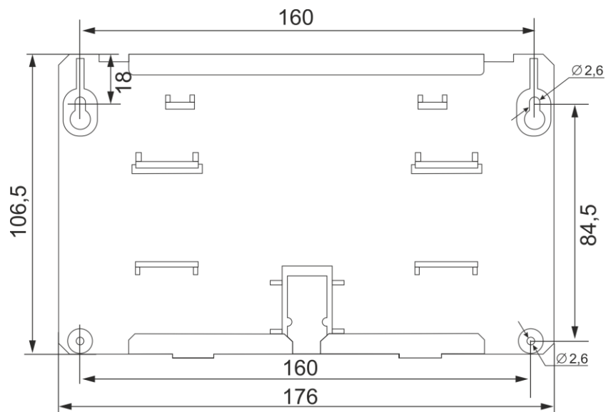
Рисунок 120. Установочный чертеж P485 и RS485/FTTx-S-SC
