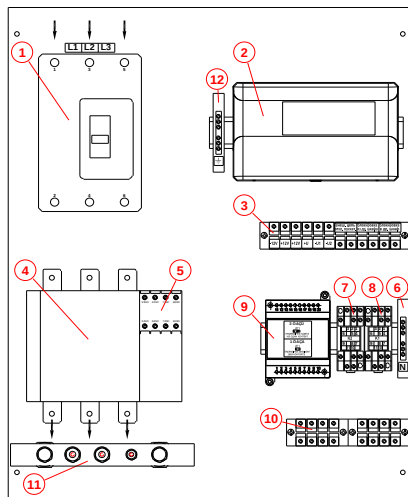
Рис. 3. Внешний вид монтажной панели исполнения ШУЭ-55-ХР777
