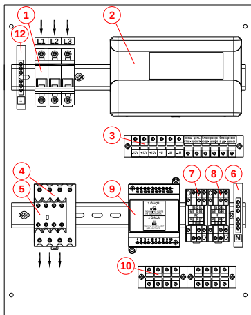
Рис. 2. Внешний вид монтажной панели исполнений ШУЭ-5,5-ХР777... ШУЭ-30-ХР777
