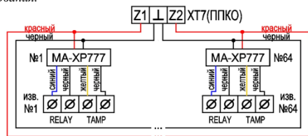
Рис. 1 Схема подключения МА-ХР777 к ШСА и извещателю
