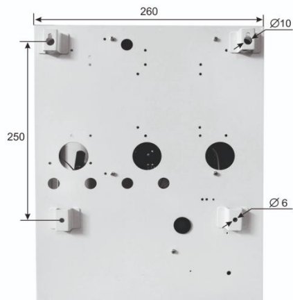
Рис. 2. Установочные размеры
