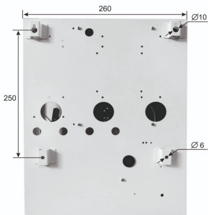
Рис. 2. Установочные размеры
