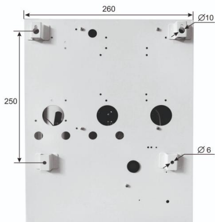
Рис. 2. Установочные размеры
