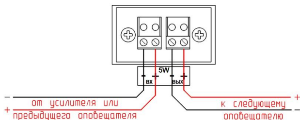
Рис. 2. Схема подключения оповещателя
