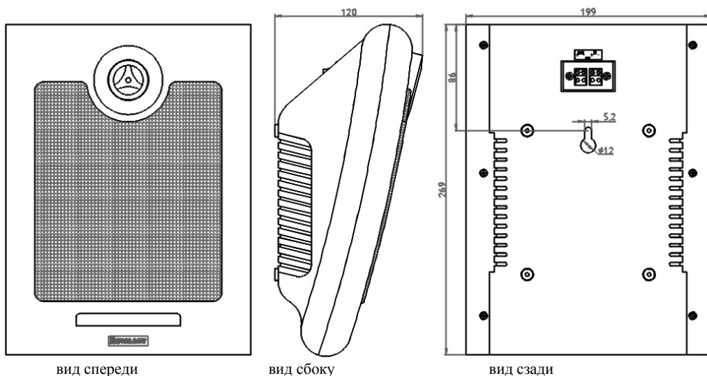
Рис. 1. Внешний вид, габаритные и установочные размеры оповещателя
