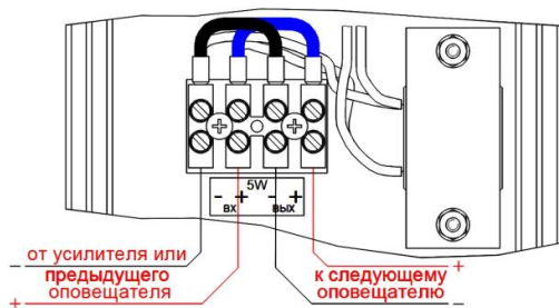
Рис. 2. Схема подключения оповещателя 5 КОМПЛЕКТНОСТЬ
