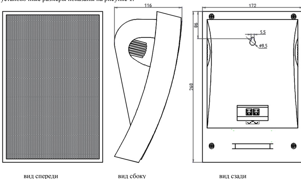
Рис. 1. Внешний вид, габаритные и установочные размеры оповещателя
