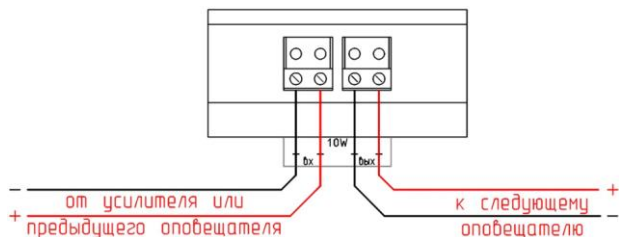
Рис. 2. Схема подключения оповещателя
