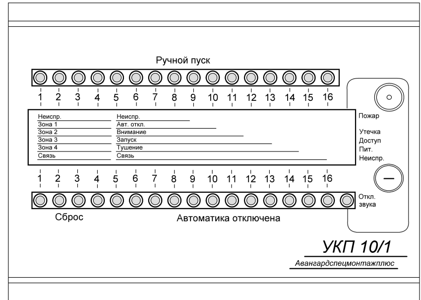
Рис. 8. Внешний вид корпуса «Березина УКП 10/1-16» модификации 4ПС
