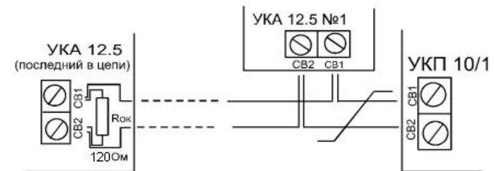
Рис.5. Последовательное подключение ППКПУ.
