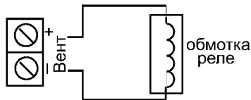
Рис.4 Схема подключения нагрузки к выходу «Вент.»
