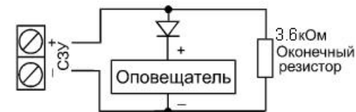
Рис.3 Схема подключения оповещателей с сопротивлением менее 300 Ом
