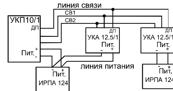
Рис.12 а) Система с отдельными блоками питания
