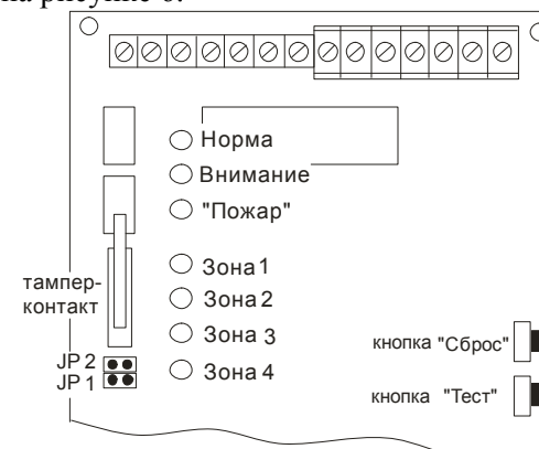
Рис.6 - Расположение светодиодов, кнопок и переключателей
