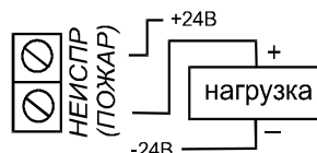
Рис.2 - Схема подключения нагрузки к выходам «Неиспр», «Пожар»
